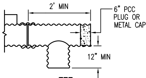
TEE
