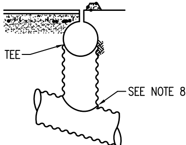
RISER
