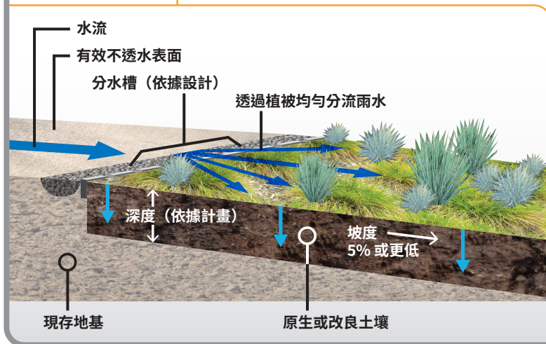
延散區（剖面圖）
